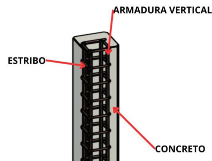
► Figura 6: Modelo de pilar de concreto
