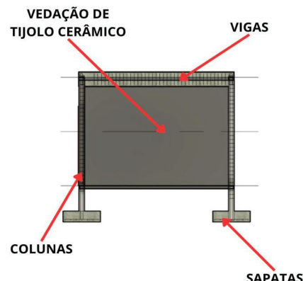
► Figura 7: Modelo de estruturas de concreto armado integrado aos outros sistemas
